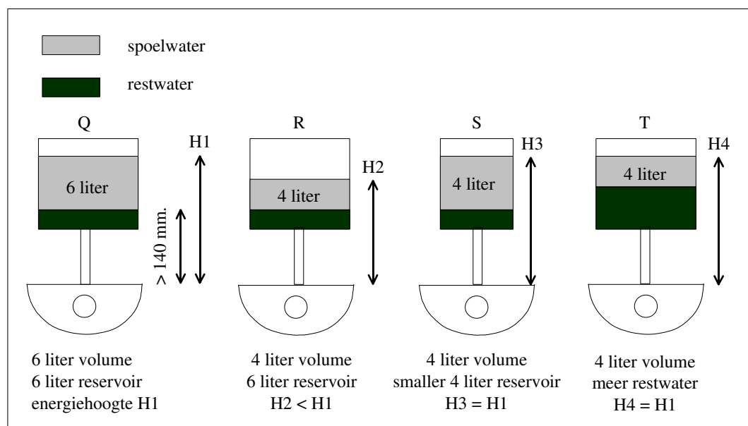
Figuur 6.4 Effect reduceren spoelvolume op energiehoogte
