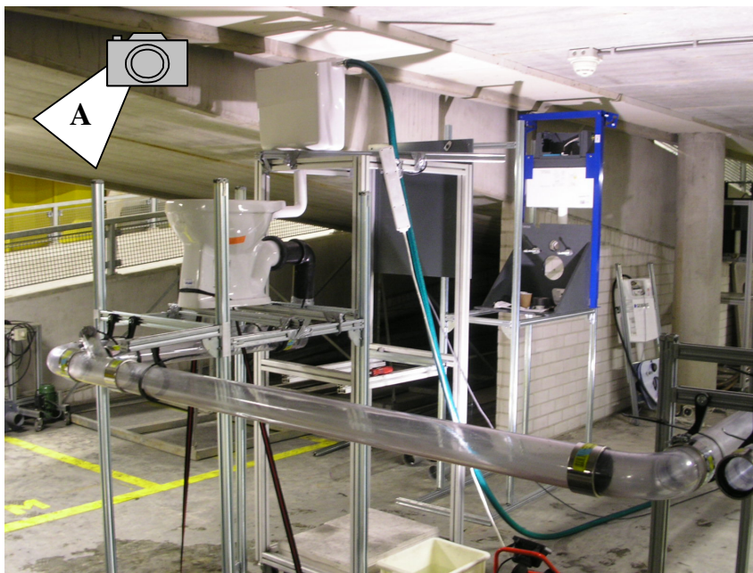
Figuur 6.2 Foto zijaanzicht meetopstelling vanaf positie A
