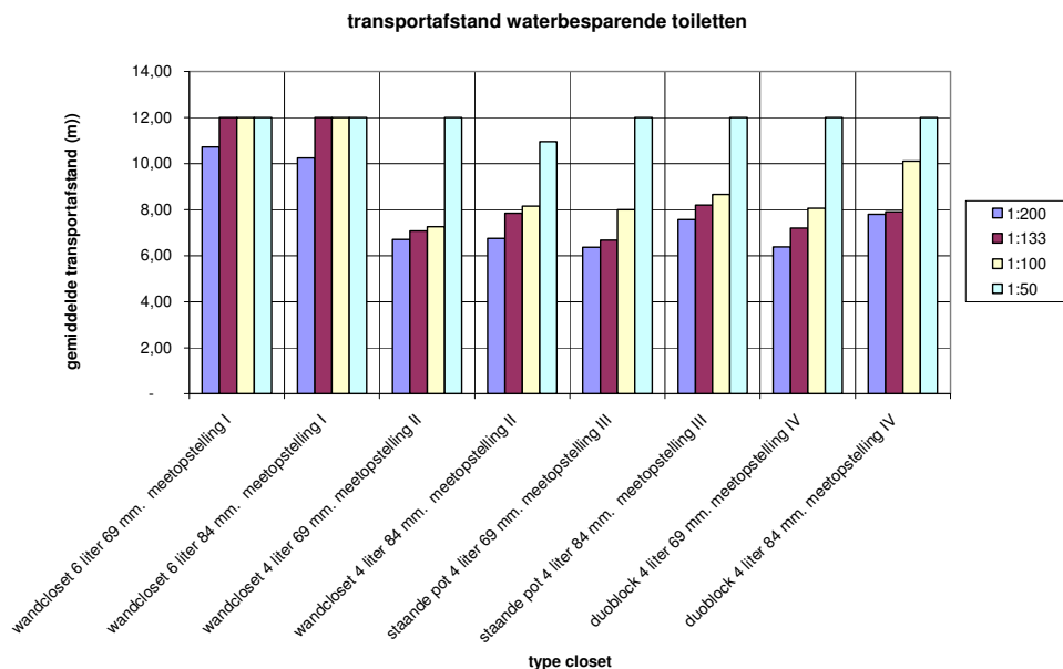
Figuur 7.1 Transportafstand na drie spoelbeurten
