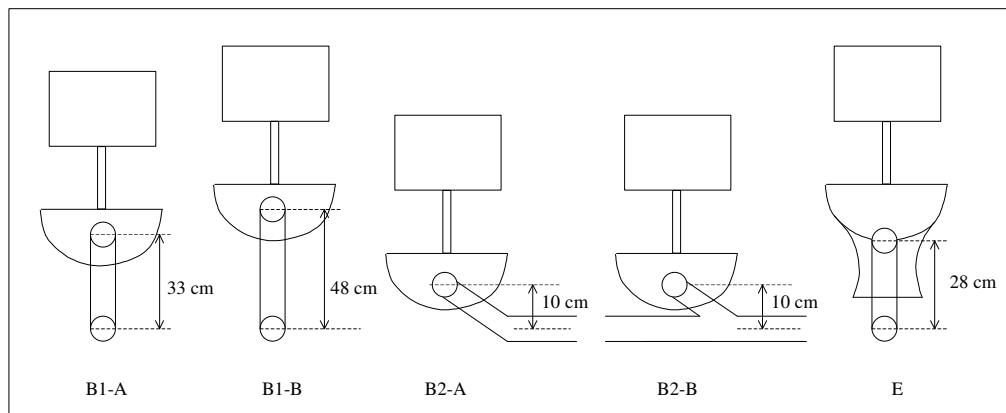
Figuur 5.1 Vijf typen wc-opstellingen
